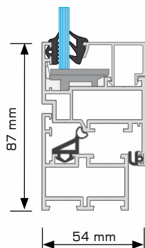
fönster i genomskärning
