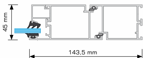
dörr i genomskärning
