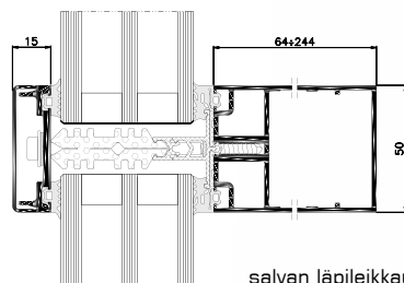
salvan läpileikkaus
